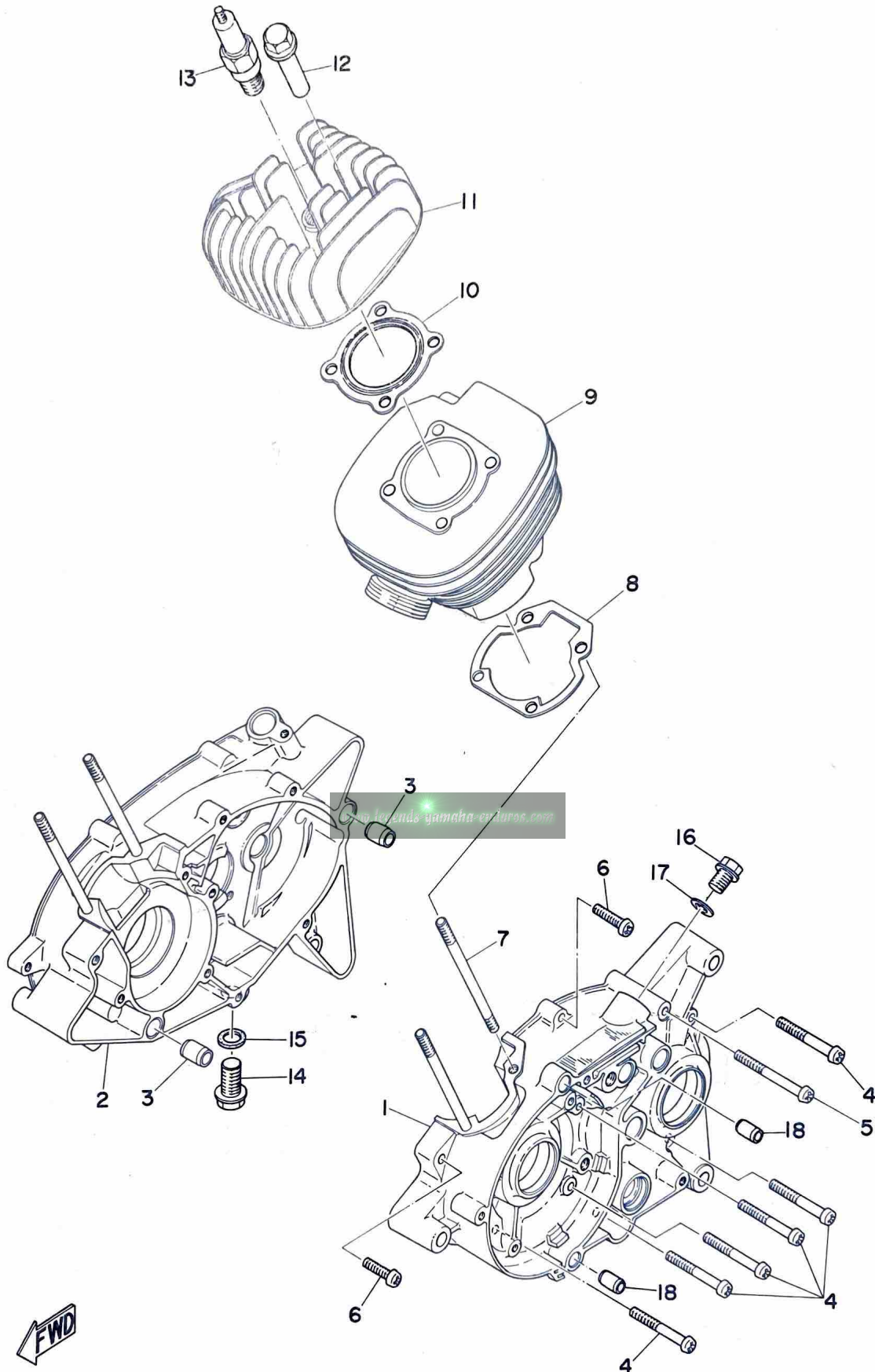
Fig. 1 CRANKCASE · CYLINDER
