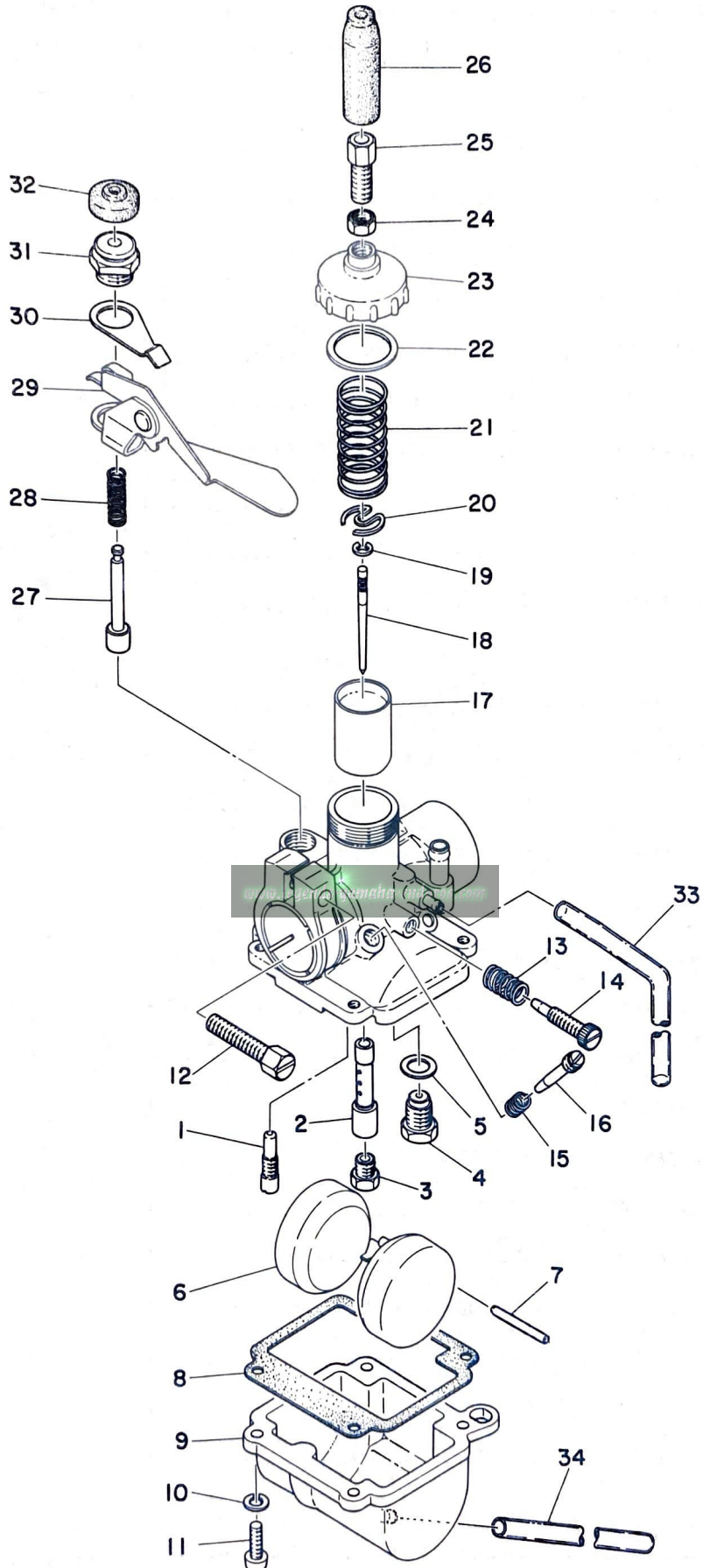
Fig. 10 CARBURETOR
