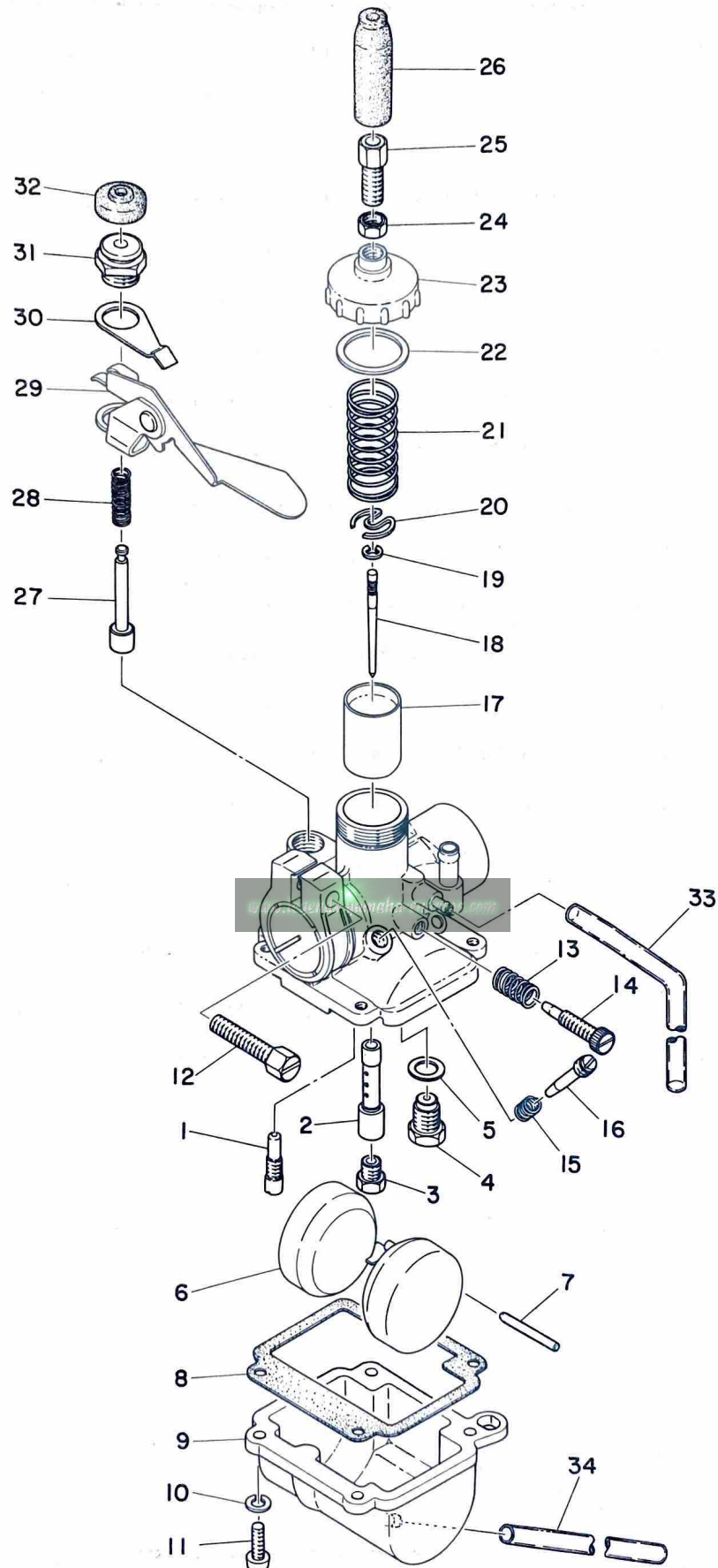
Fig. 10 CARBURETOR
