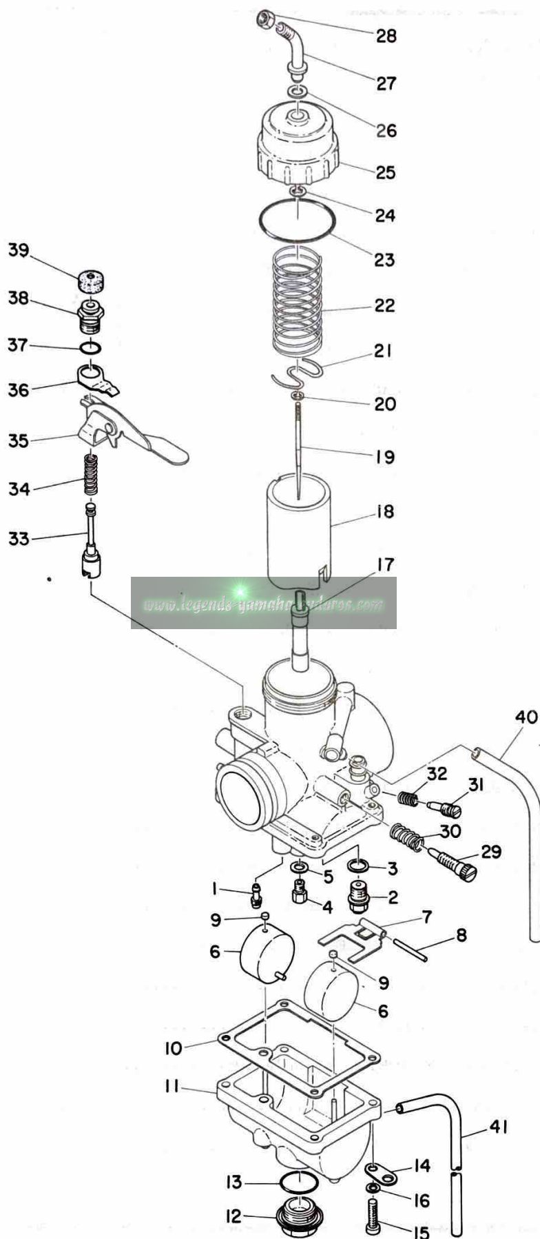
Fig. 14 CARBURETOR (DT400B)
