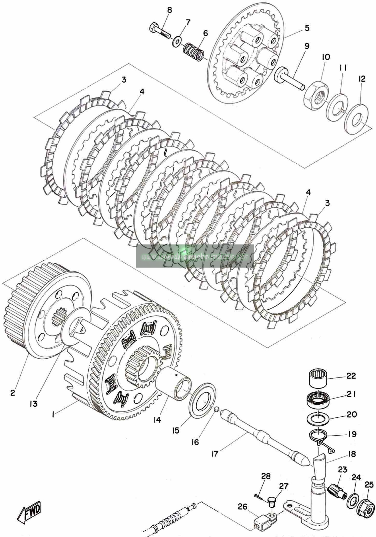
Fig. 5 CLUTCH
