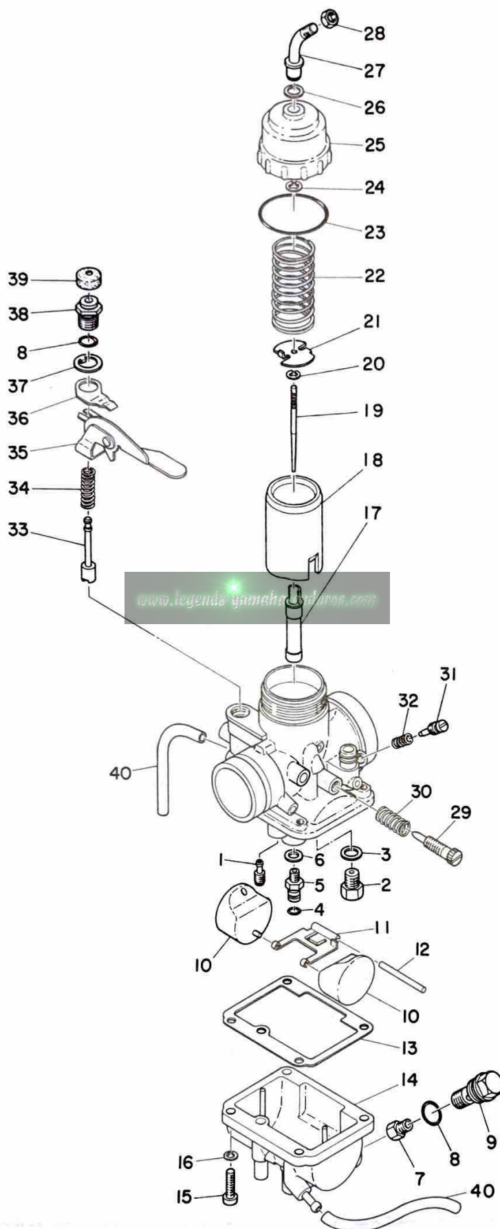
Fig. 13 CARBURETOR (DT250B)
