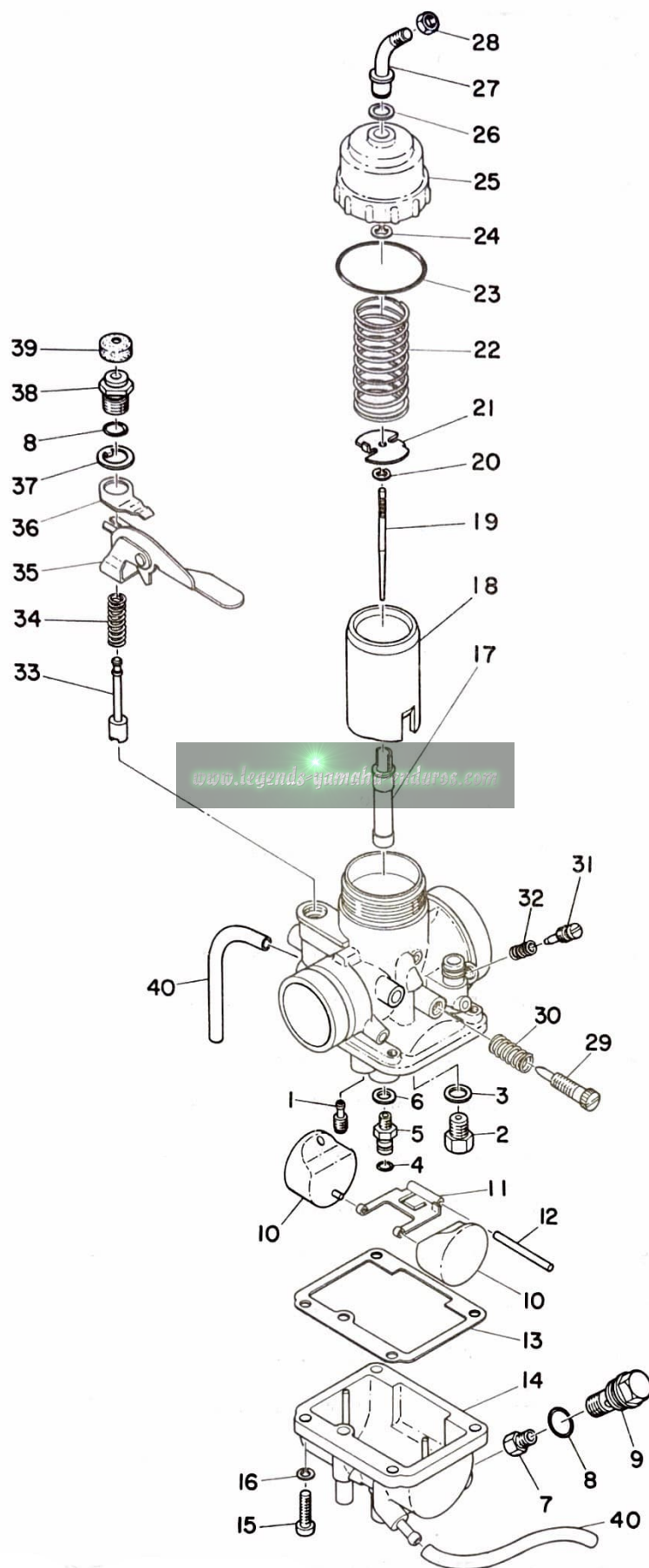
Fig. 13 CARBURETOR (DT250B)
