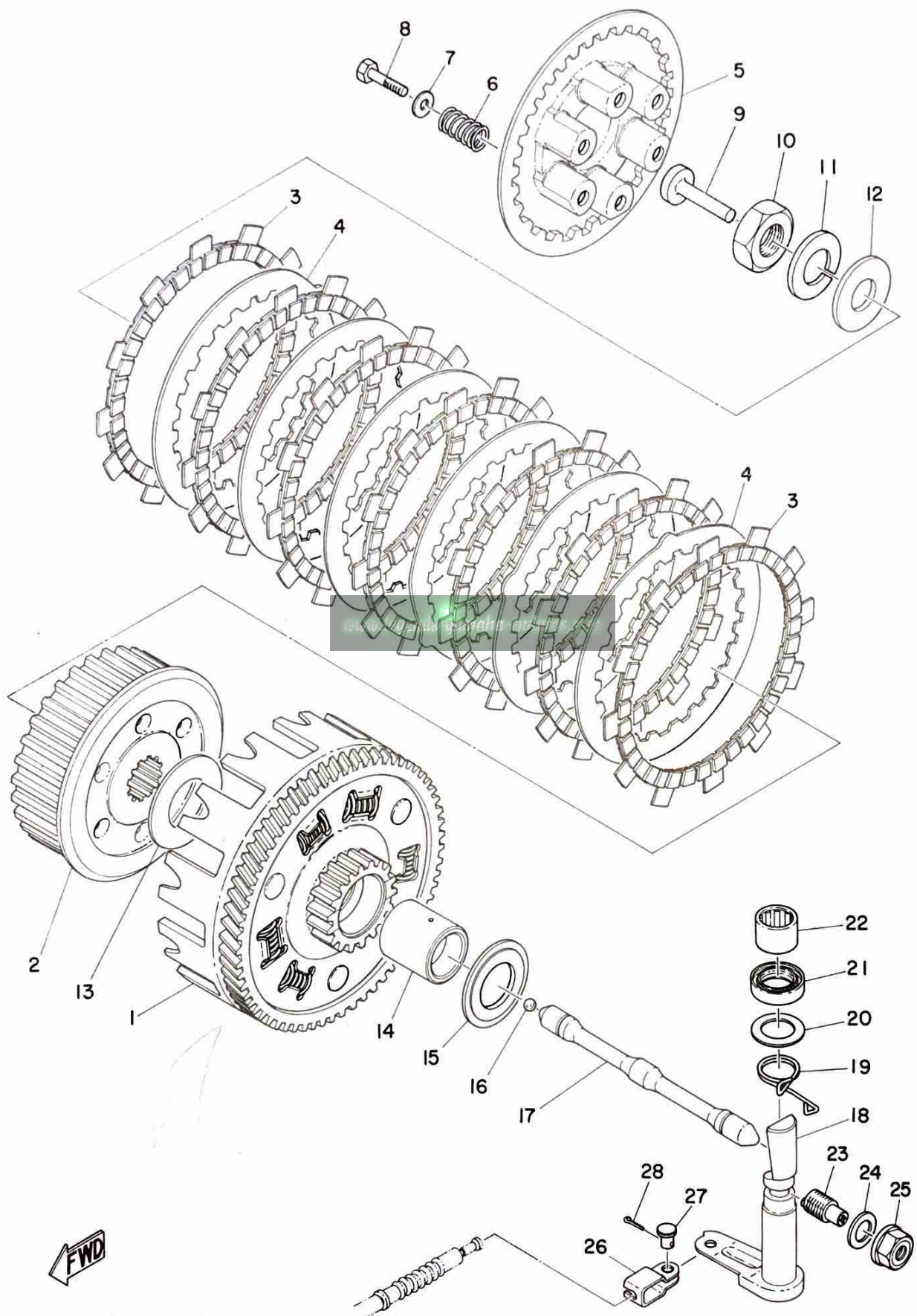
Fig. 5 CLUTCH
