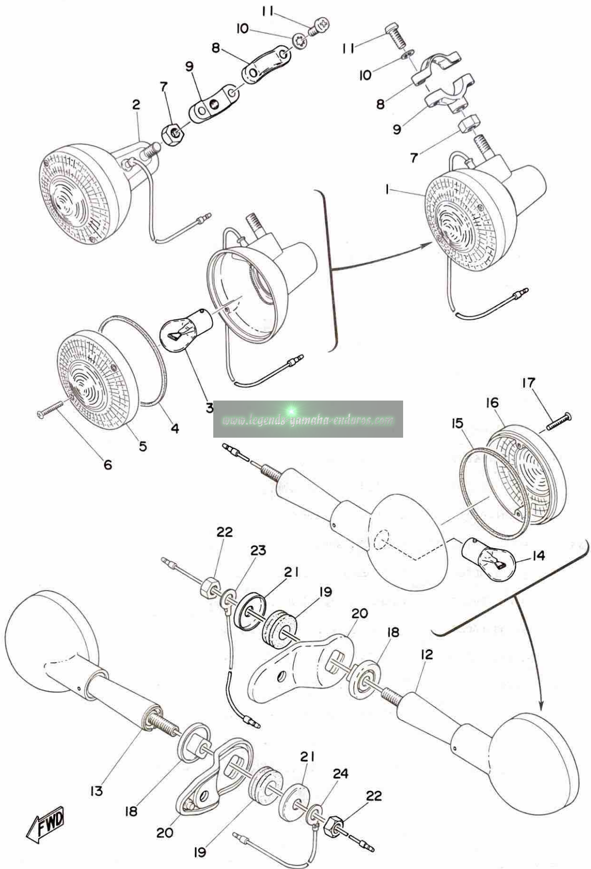
Fig. 34 FLASHER LAMP
