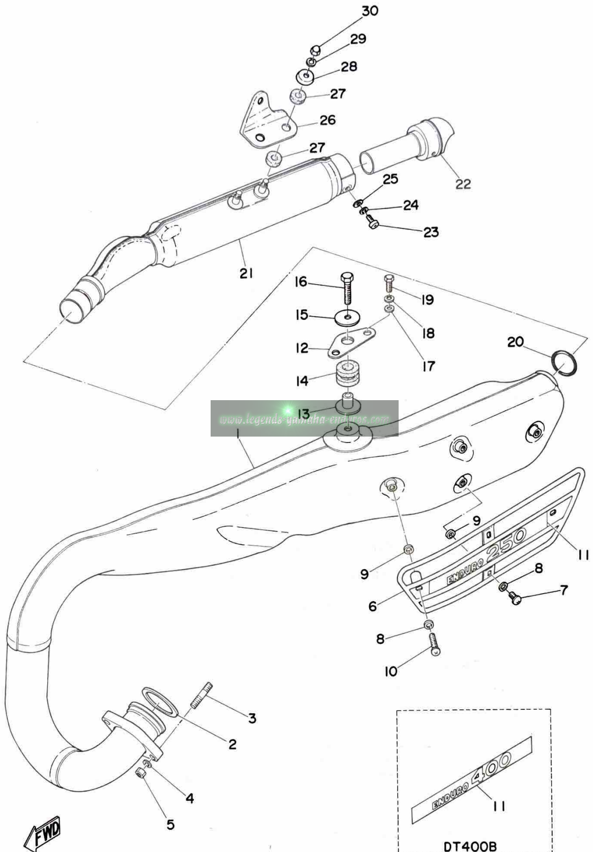
Fig. 15 EXHAUST
