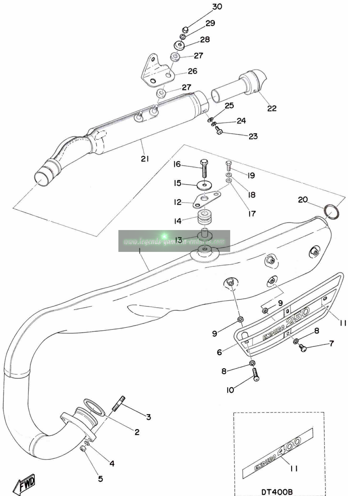
Fig. 15 EXHAUST
