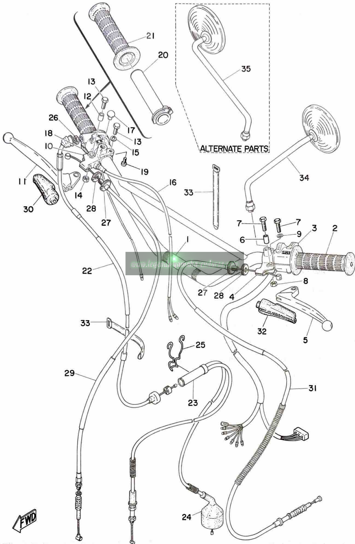
Fig. 25 HANDLE · WIRE
