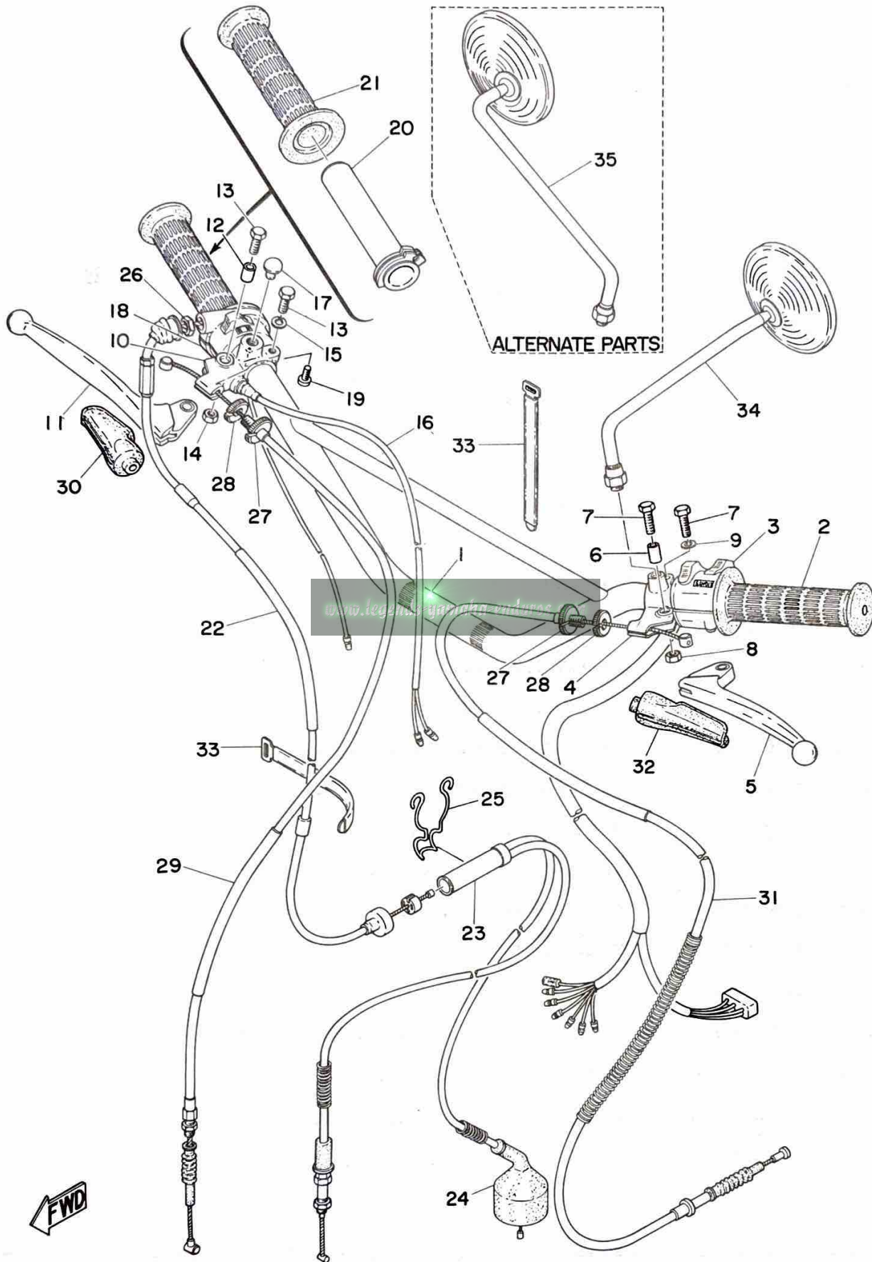
Fig. 25 HANDLE · WIRE
