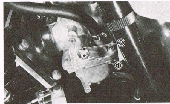
1. Throttle stop screw 1. Vis butée d'accélérateur 2. Lock nut 2. Ecrou de blocage
