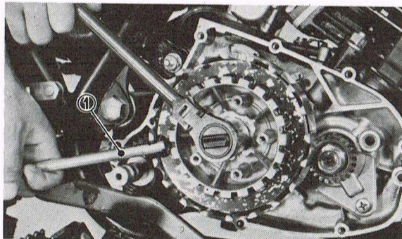
1. Outil de maintien d'embrayage
