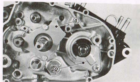
1. Bearing cover plate 1. Plaque de retenue du roulement 2. Oil seal holder 2. Retenue du renvoi d'huile
