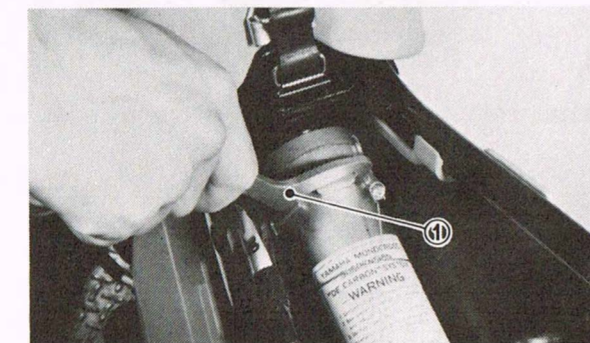
1. Special nut wrench 1. Clé pour écrou spécial
