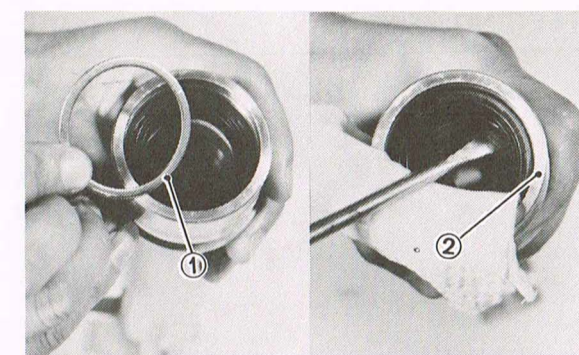
1. Washer 2. Oil seal 1. Rondelle 2. Bague d'étanchéité
