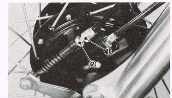
1. Adjuster 1. Dispositif de réglage 2. Lock nut 2. Ecrou de blocage
