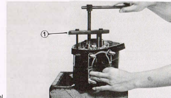
1. Outil de séparation du carter
