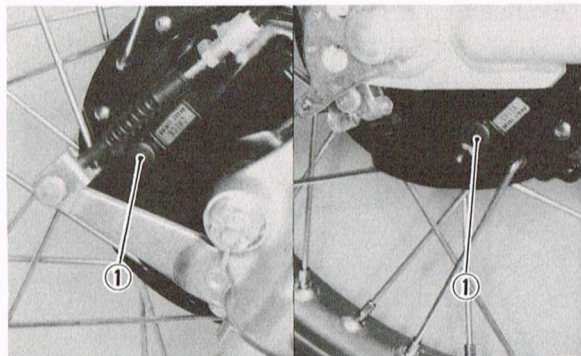
1. Inspection hole 1. Contrôle de trou
