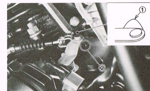
1. Push lever mark 1. Repère du levier 2. Case match mark 2. Repère du carter d'alignement
