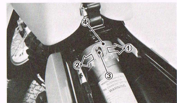
1. Stiffer 2. Softer 3. Adjuster stopper 4. Adjuster 1. Ressort devient plus dur 2. Ressort devient plus souple 3. Arrêteur du siège du ressort 4. Einstellschraube
