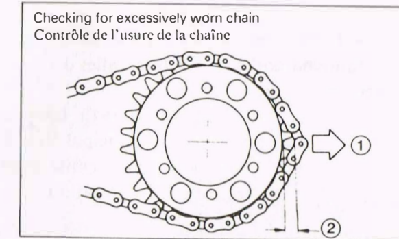
1. Pull 2. 1/2 teeth
