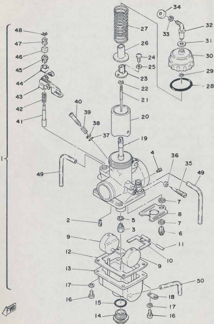
Fig. 10 CARBURETOR
