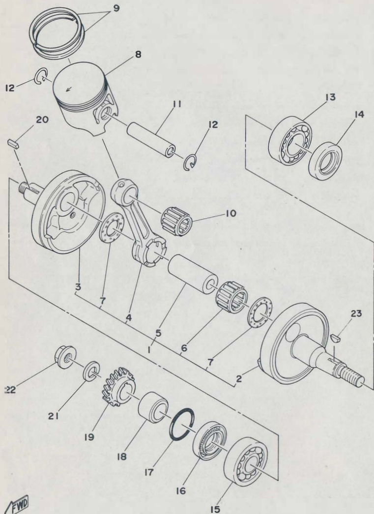
Fig. 3 CRANK · PISTON
