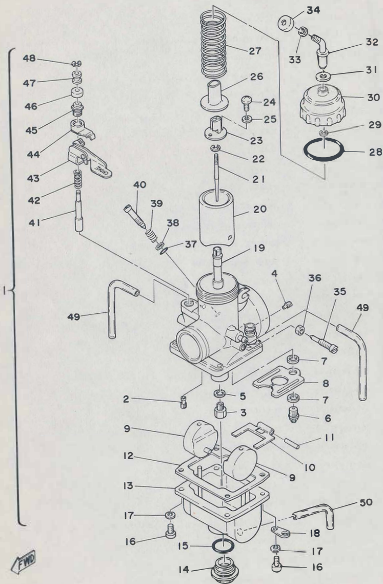
Fig. 10 CARBURETOR
