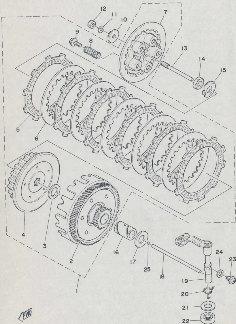
Fig. 4 CLUTCH
