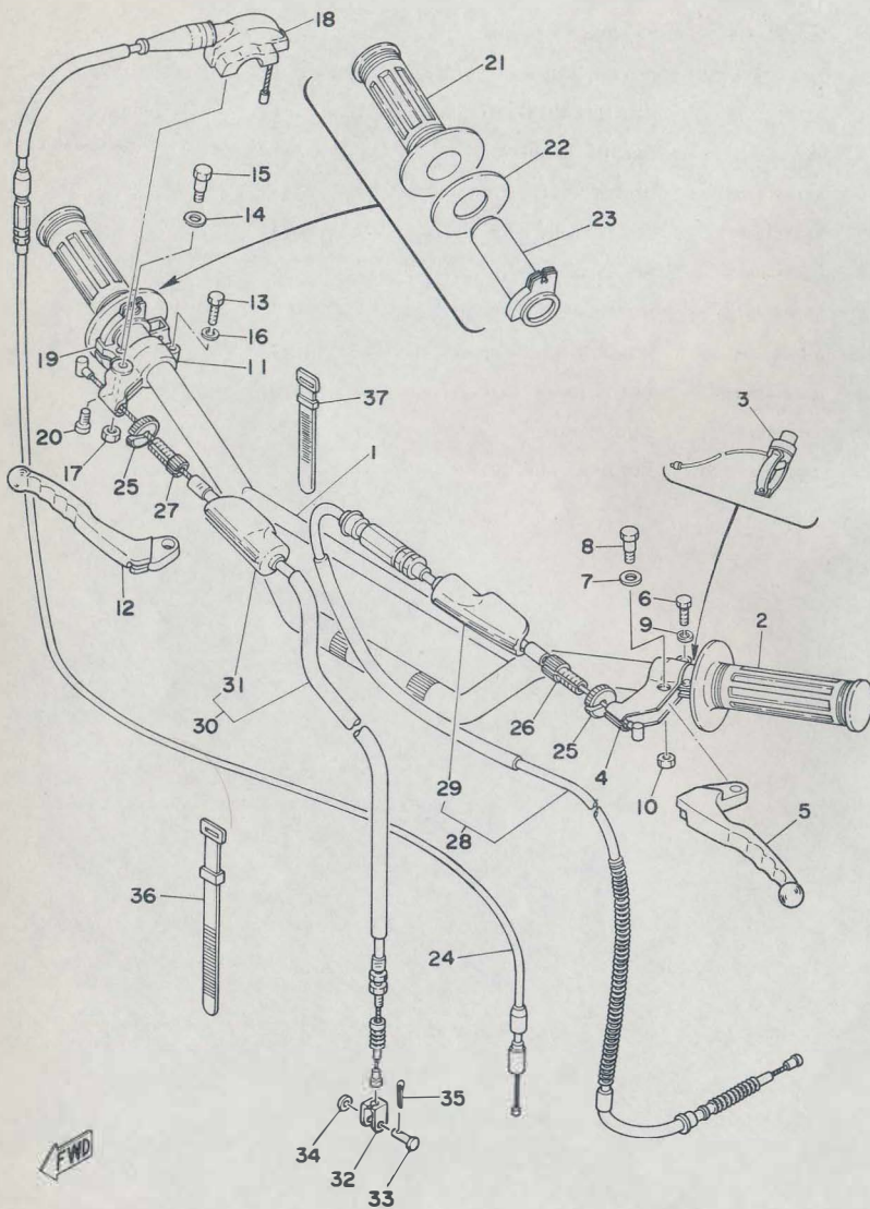
Fig. 22 HANDLE · WIRE
