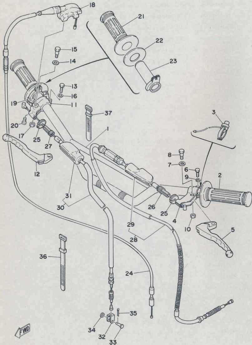
Fig. 22 HANDLE · WIRE
