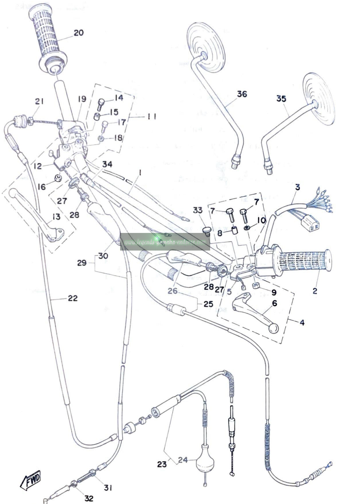
Fig. 21 HANDLE · WIRE
