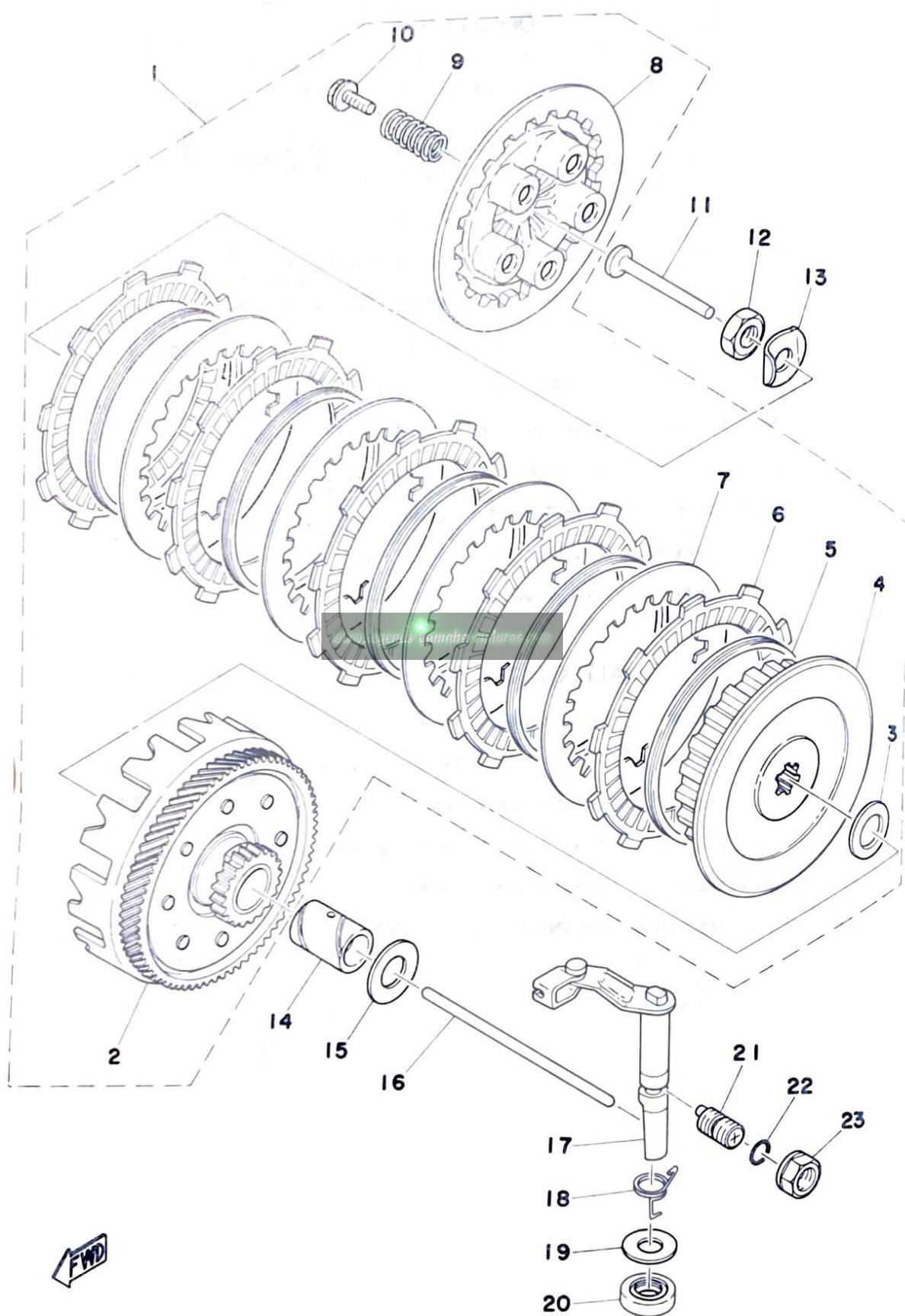
Fig. 4 CLUTCH
