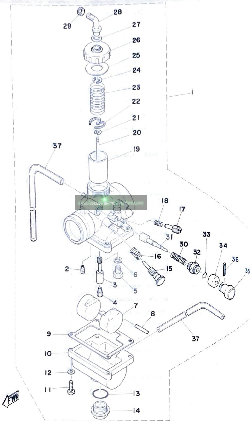
Fig. 11 CARBURETOR
