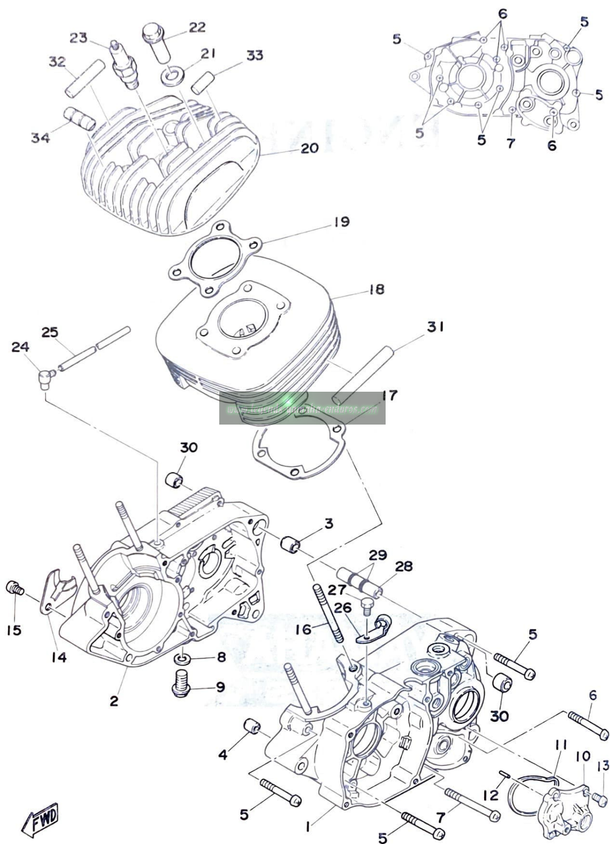
Fig. 1 CRANKCASE · CYLINDER
