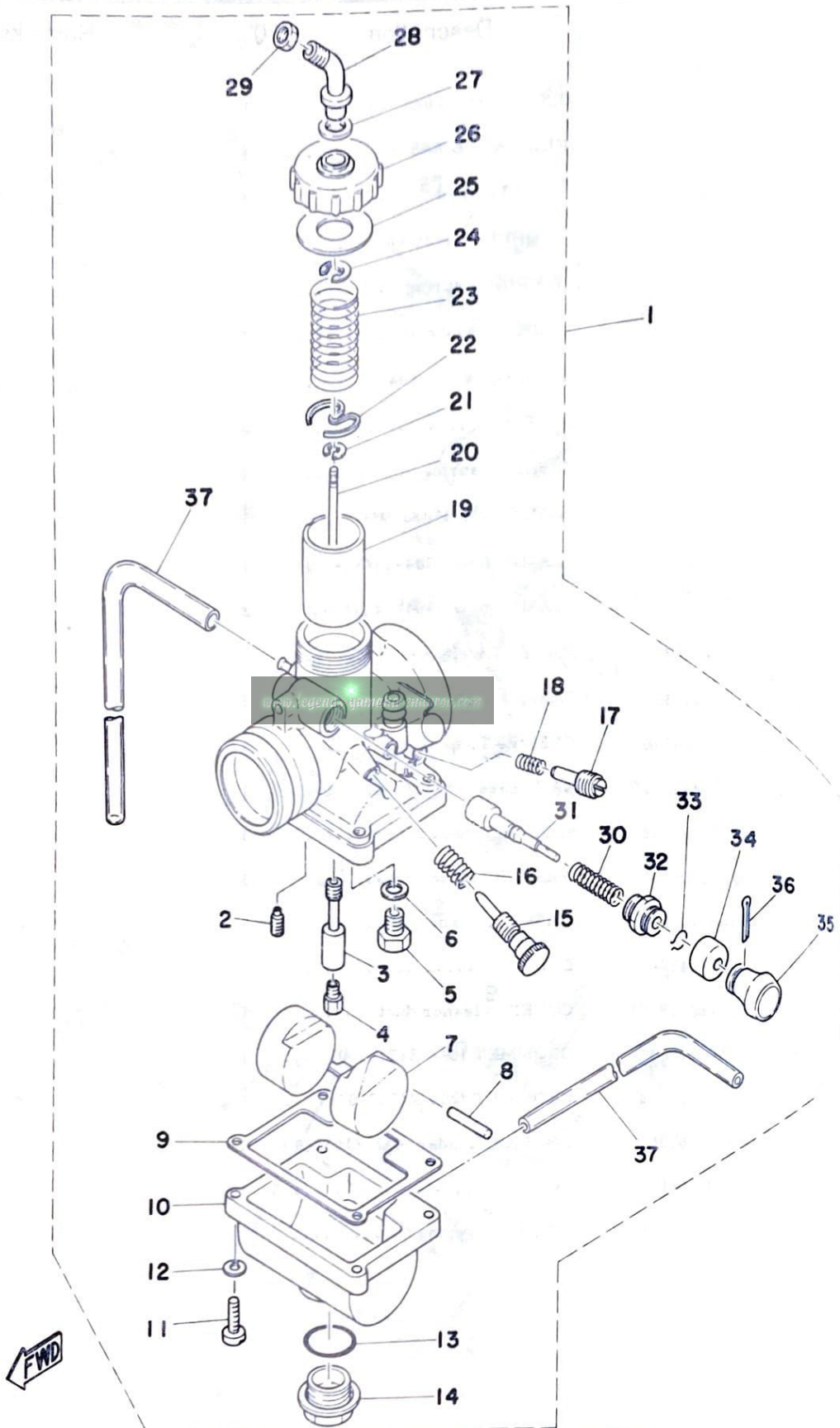
Fig. 11 CARBURETOR
