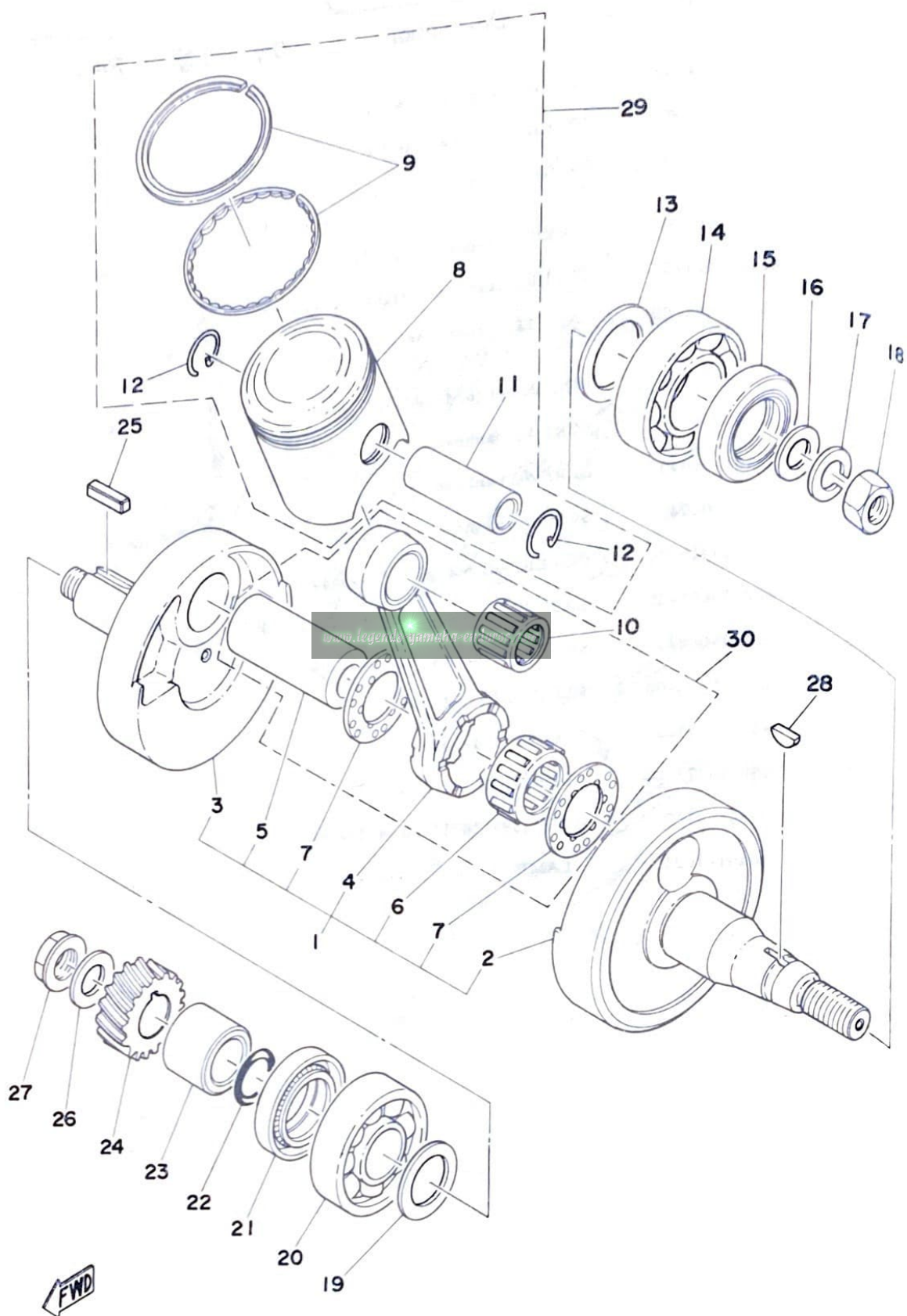
Fig. 3 CRANK · PISTON
