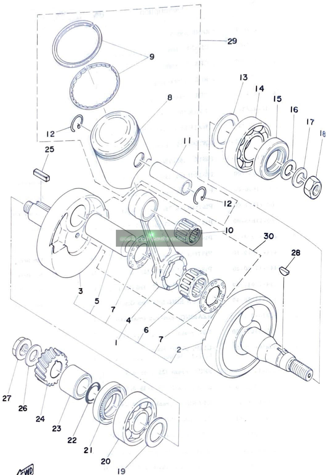
Fig. 3 CRANK · PISTON
