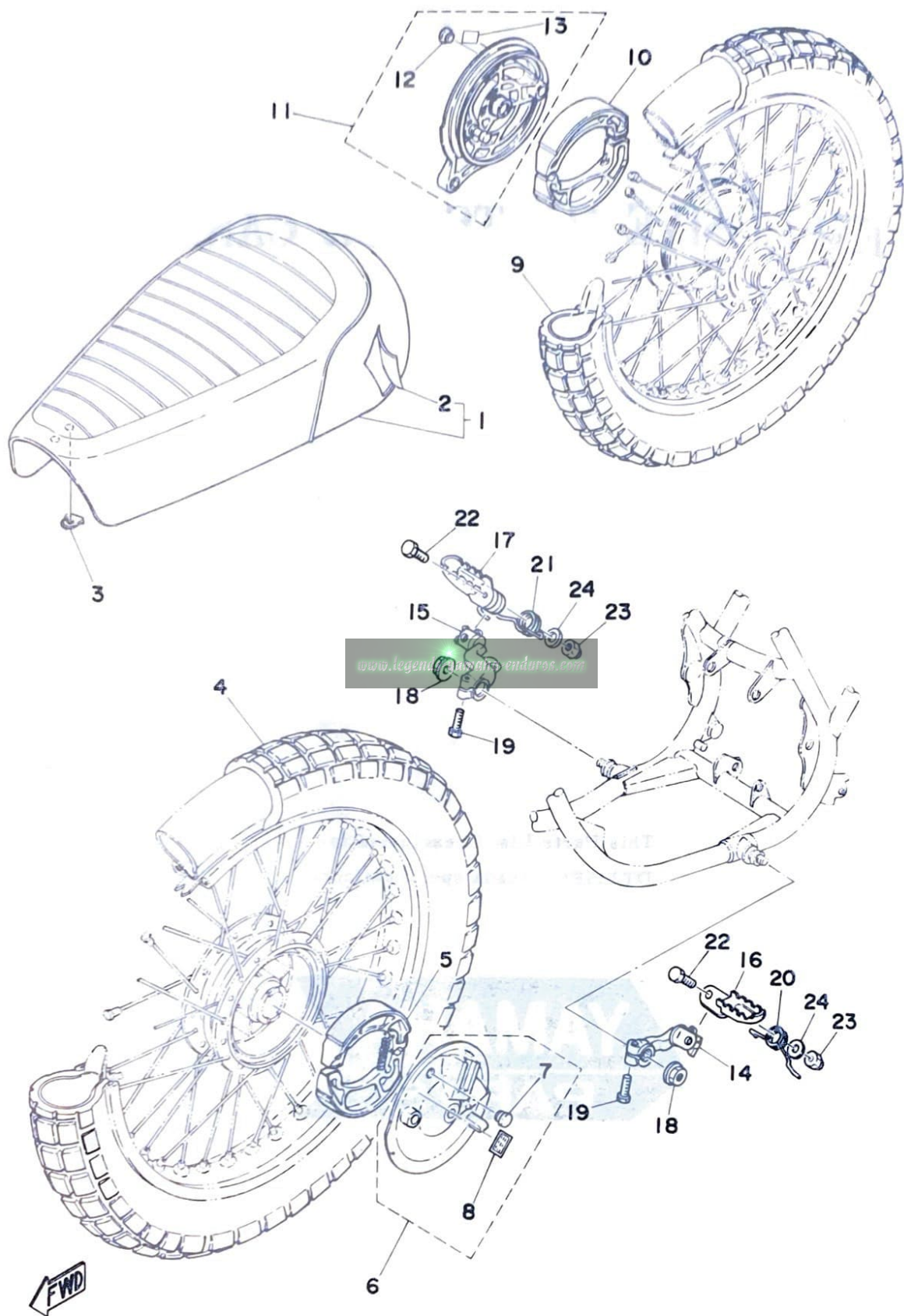
Fig. 32 SEAT · WHEEL
