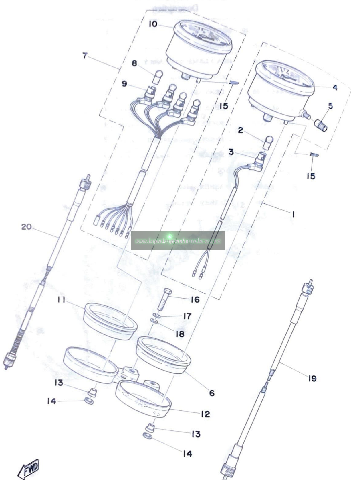
Fig. 28 SPEEDOMETER · TACHOMETER
