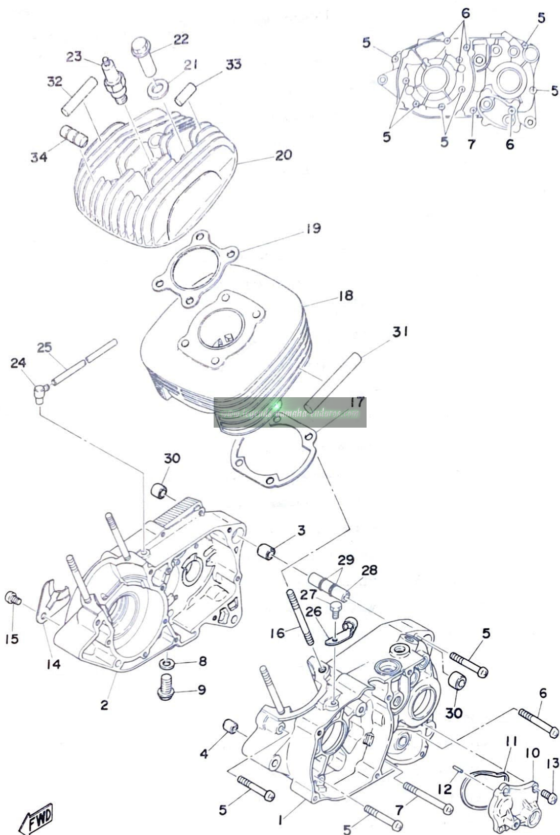
Fig. 1 CRANKCASE · CYLINDER
