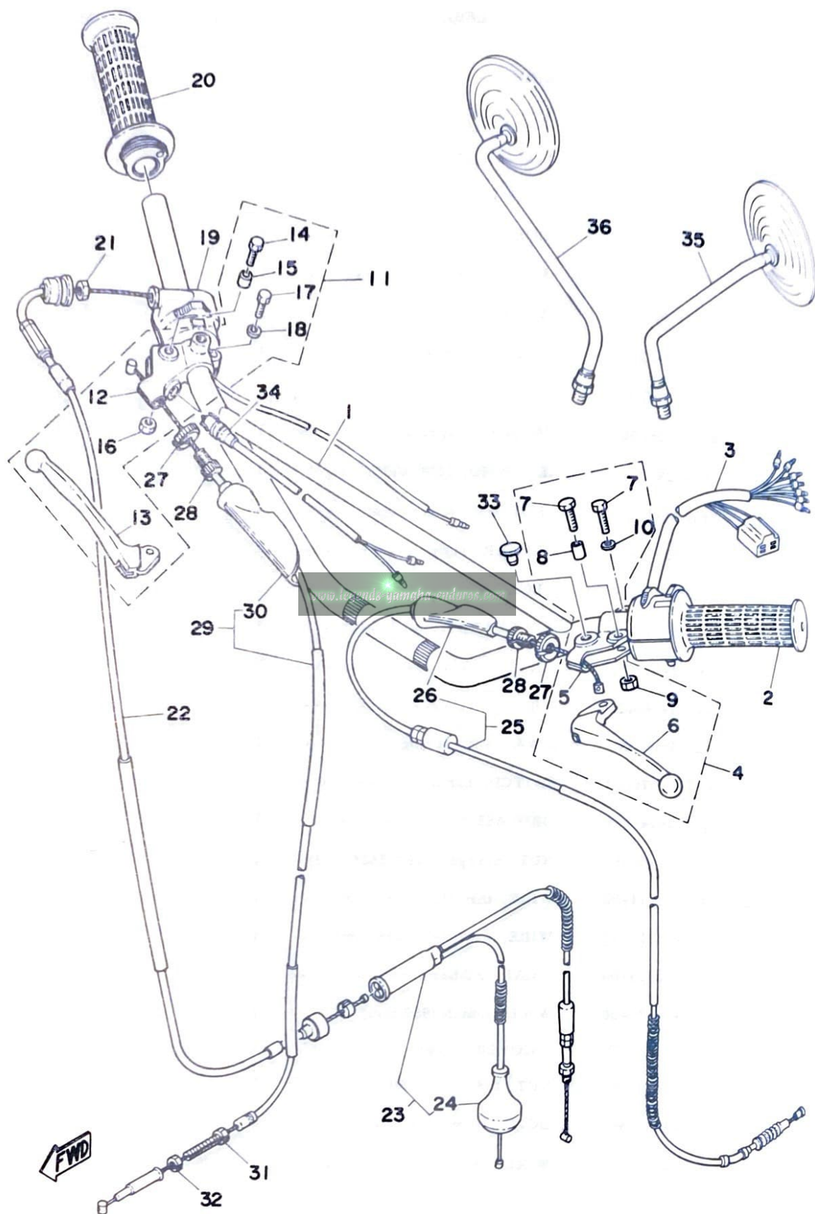
Fig. 21 HANDLE · WIRE
