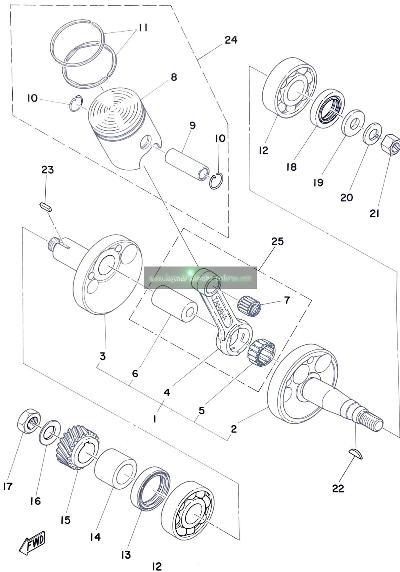
Fig. 3 CRANK · PISTON
