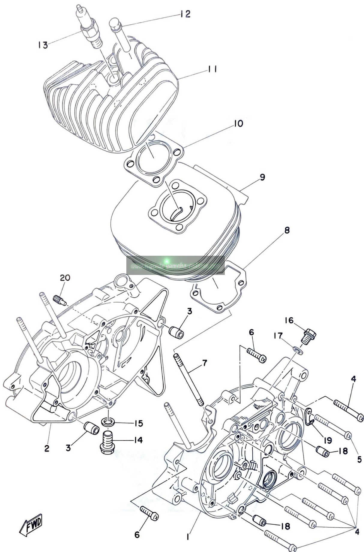
Fig. 1 CRANKCASE · CYLINDER
