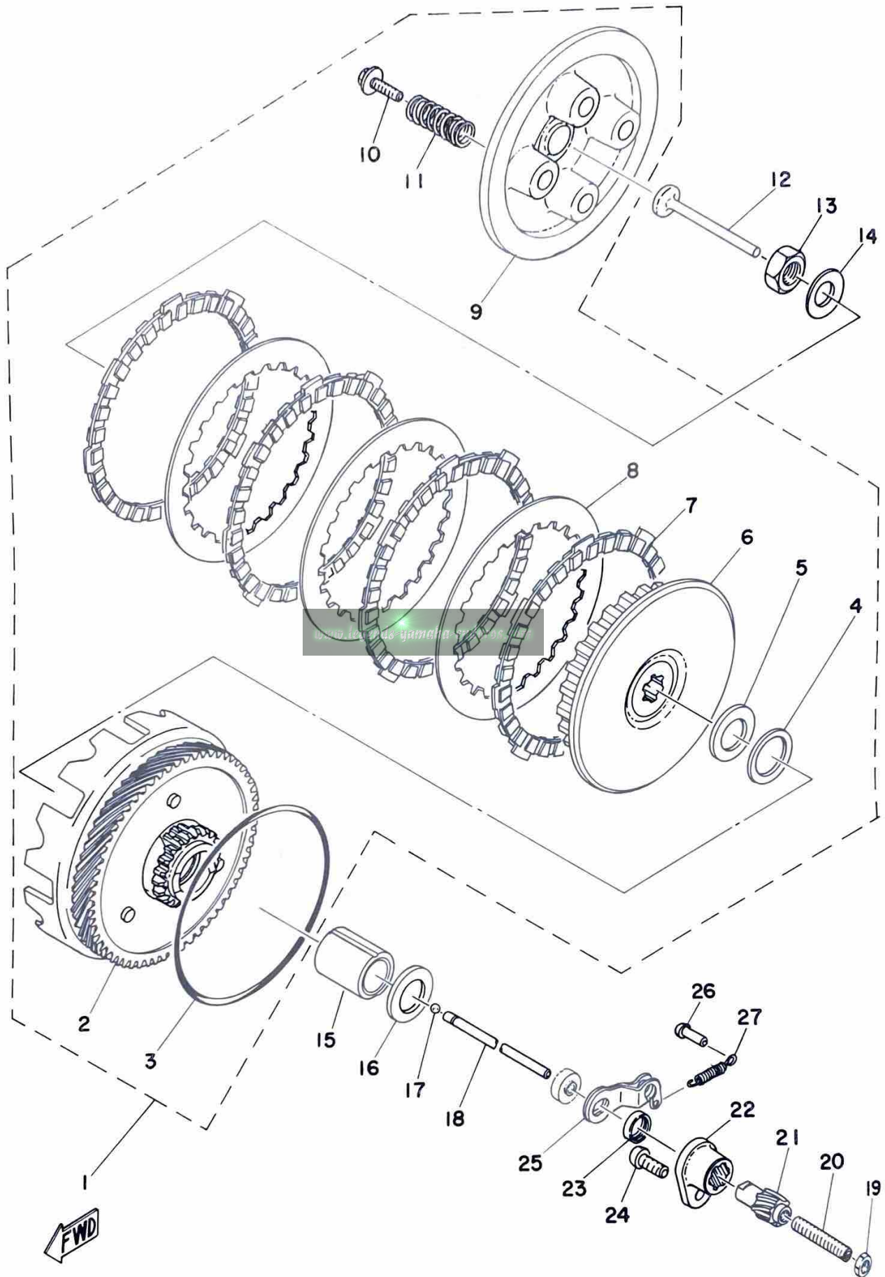
Fig. 4 CLUTCH
