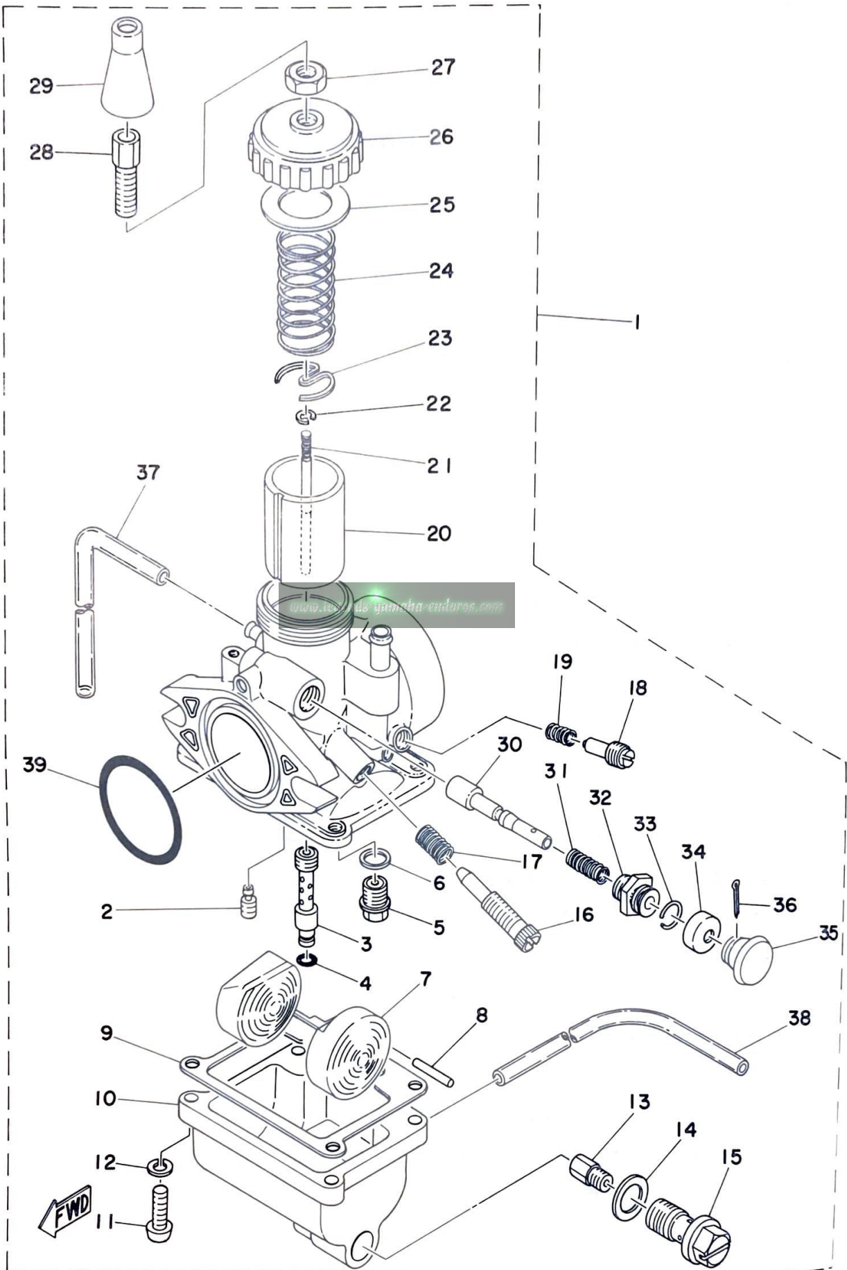
Fig. 10 CARBURETOR
