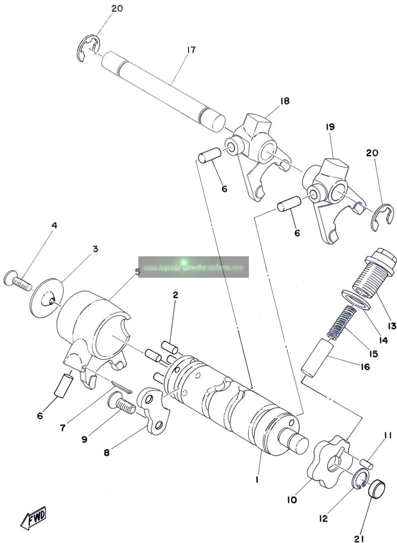
Fig. 6 SHIFTER 1
