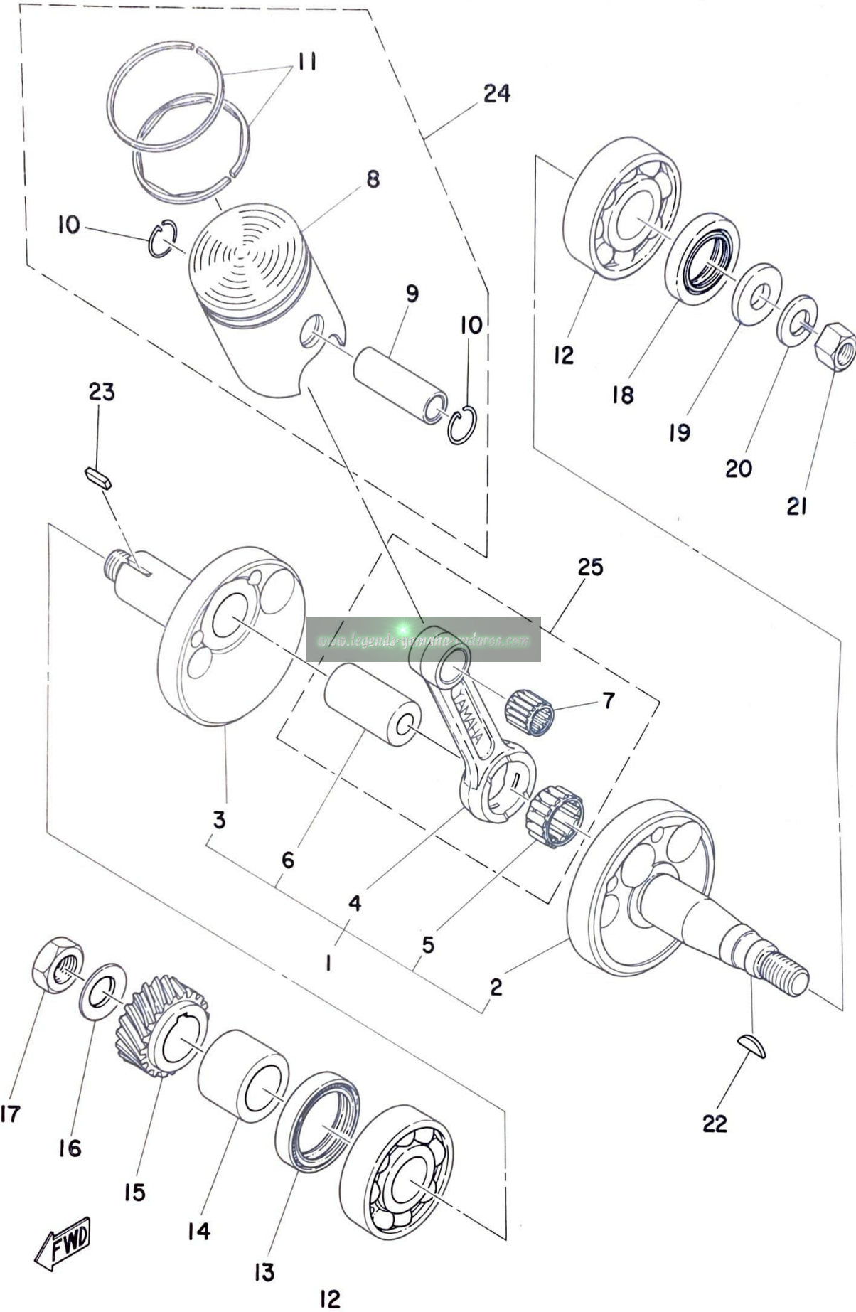
Fig. 3 CRANK · PISTON
