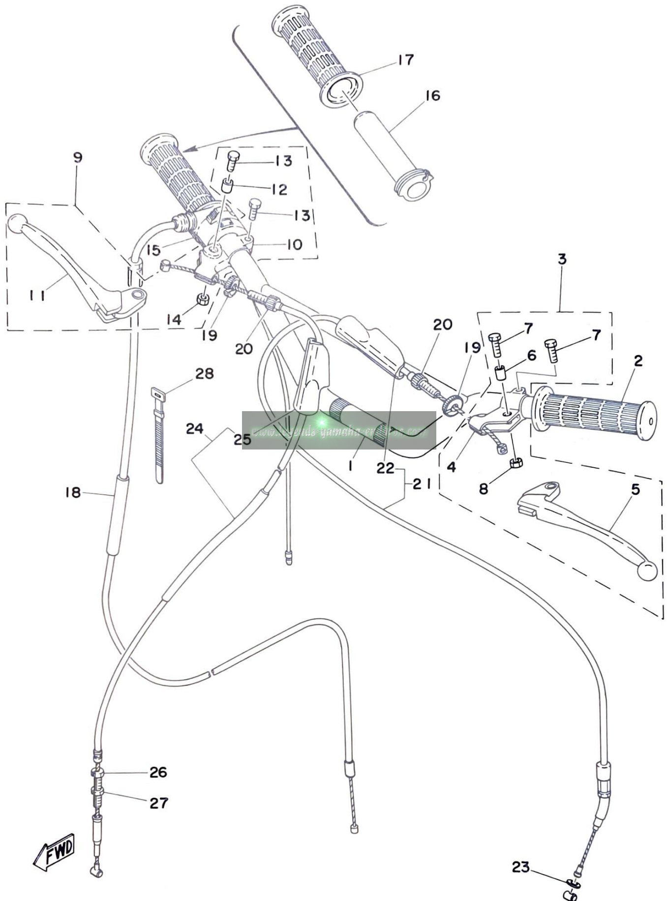
Fig. 19 HANDLE · WIRE
