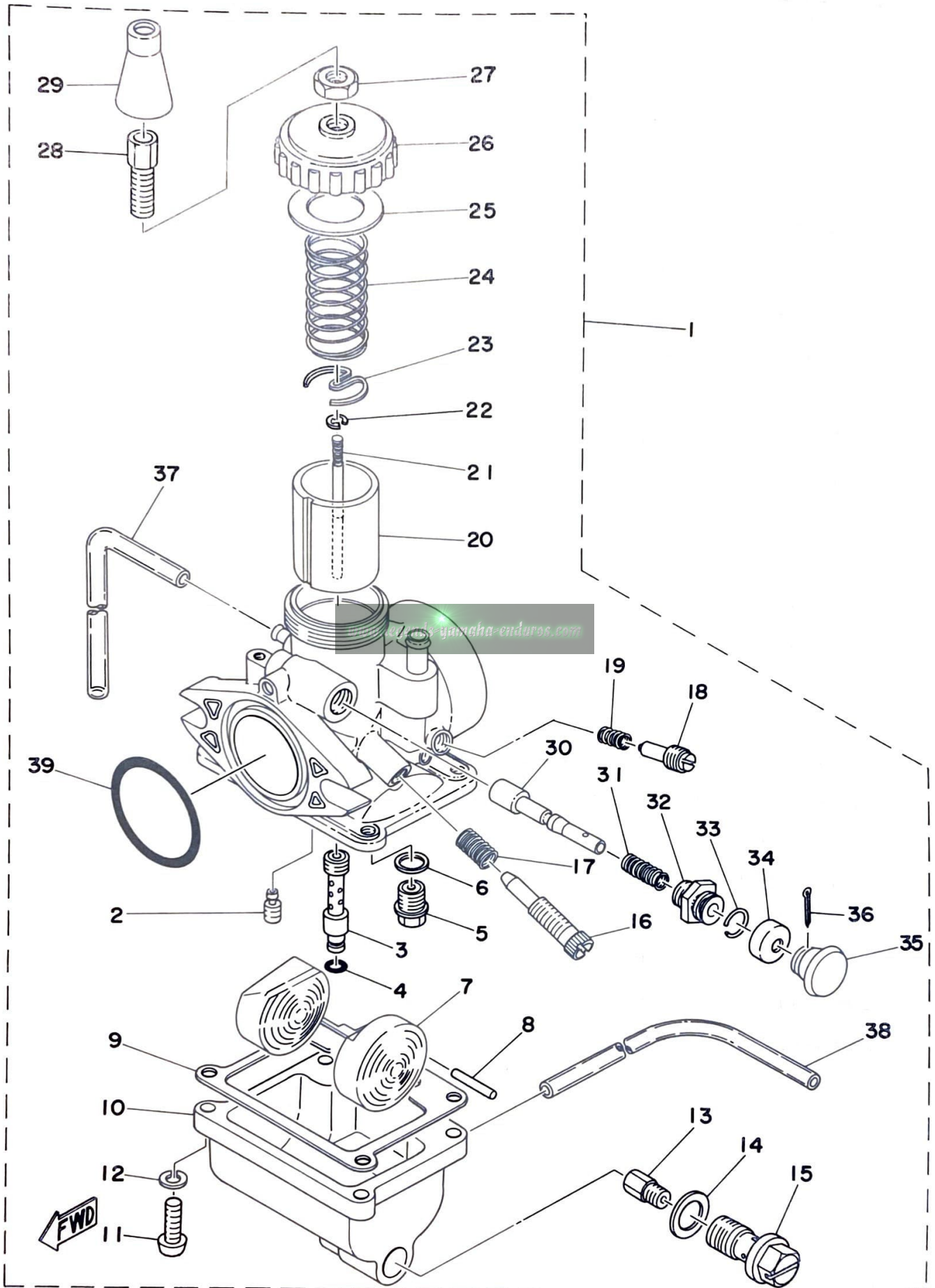
Fig. 10 CARBURETOR
