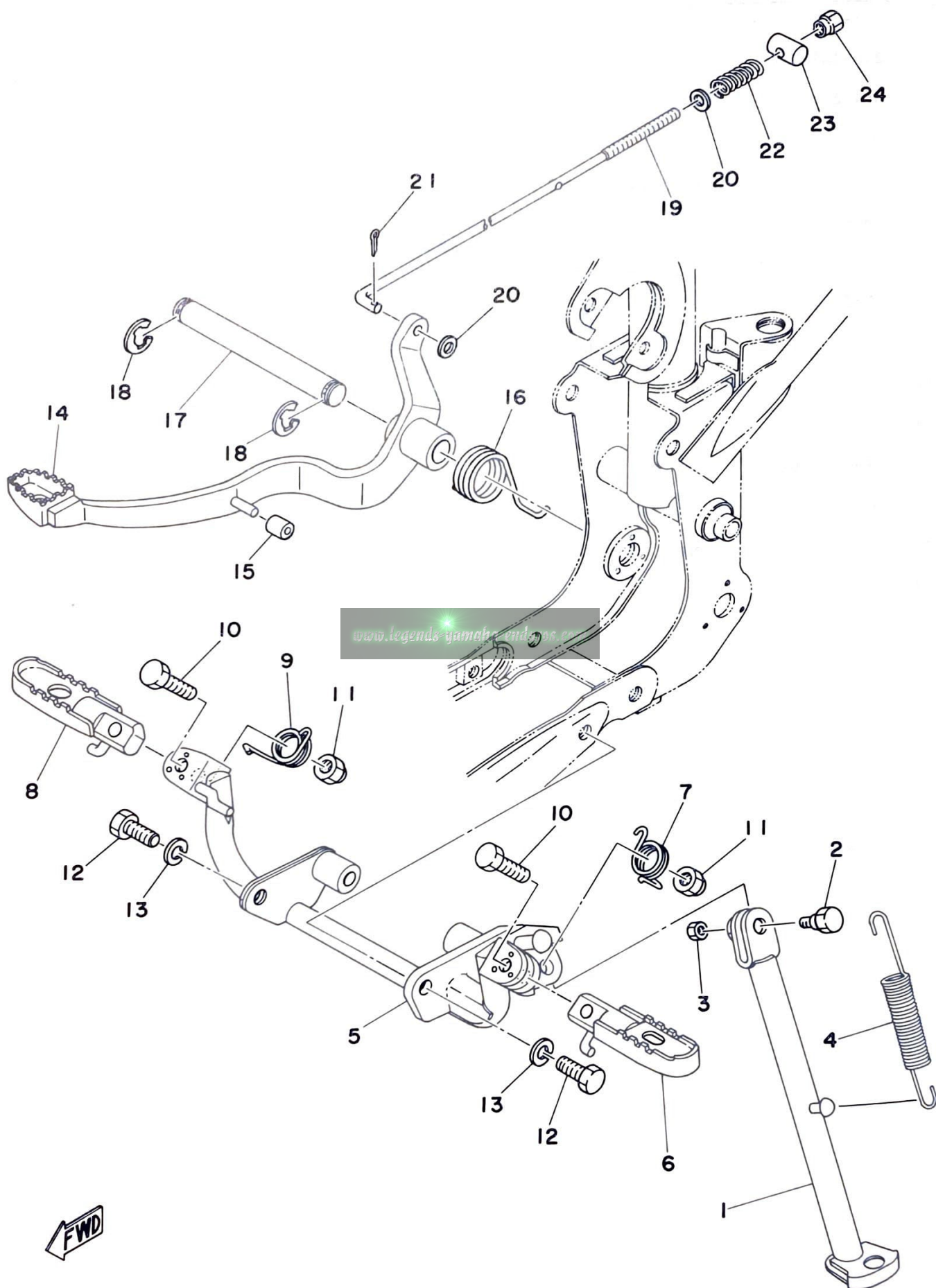
Fig. 15 STAND · FOOTREST · BRAKE PEDAL
