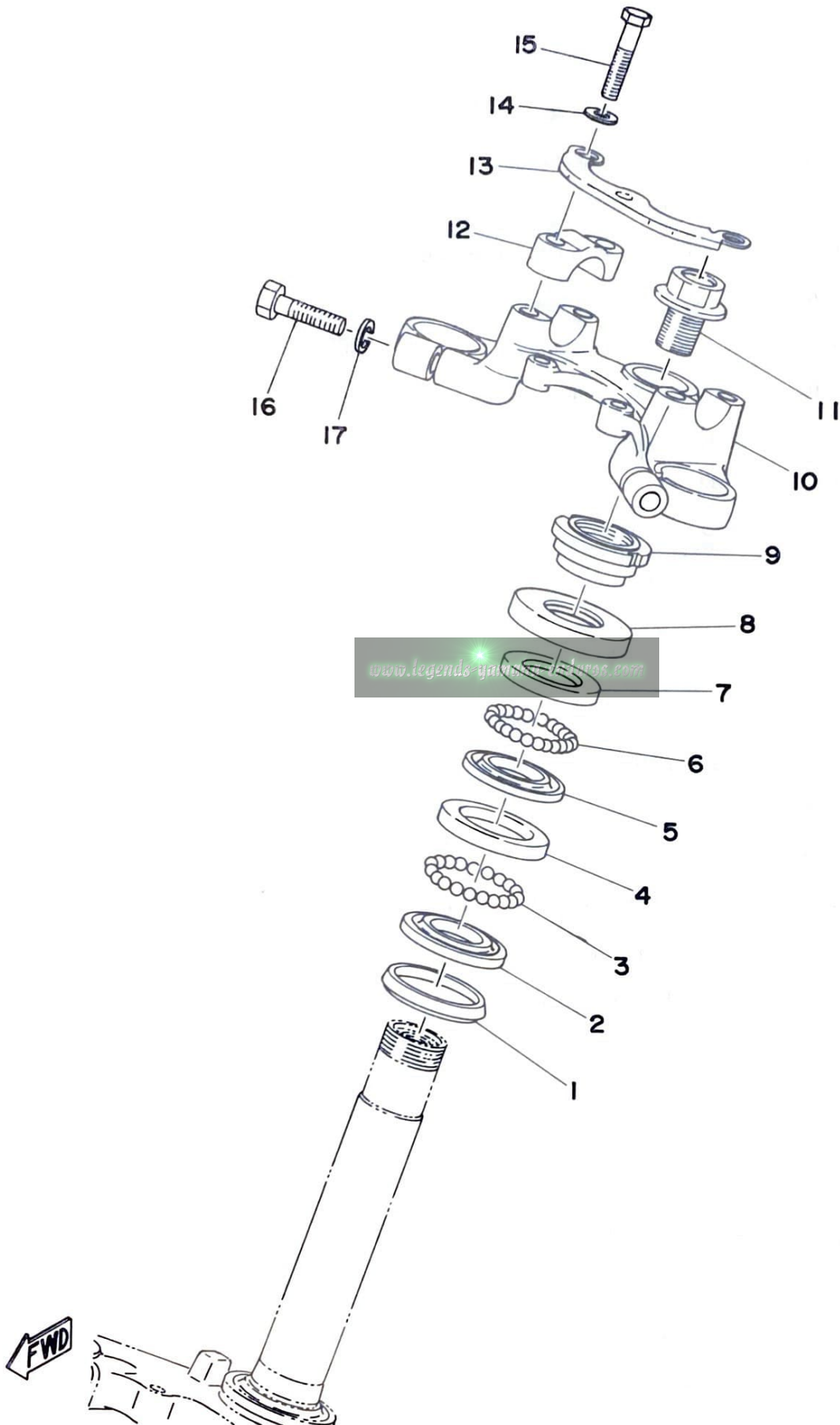
Fig. 18 STEERING
