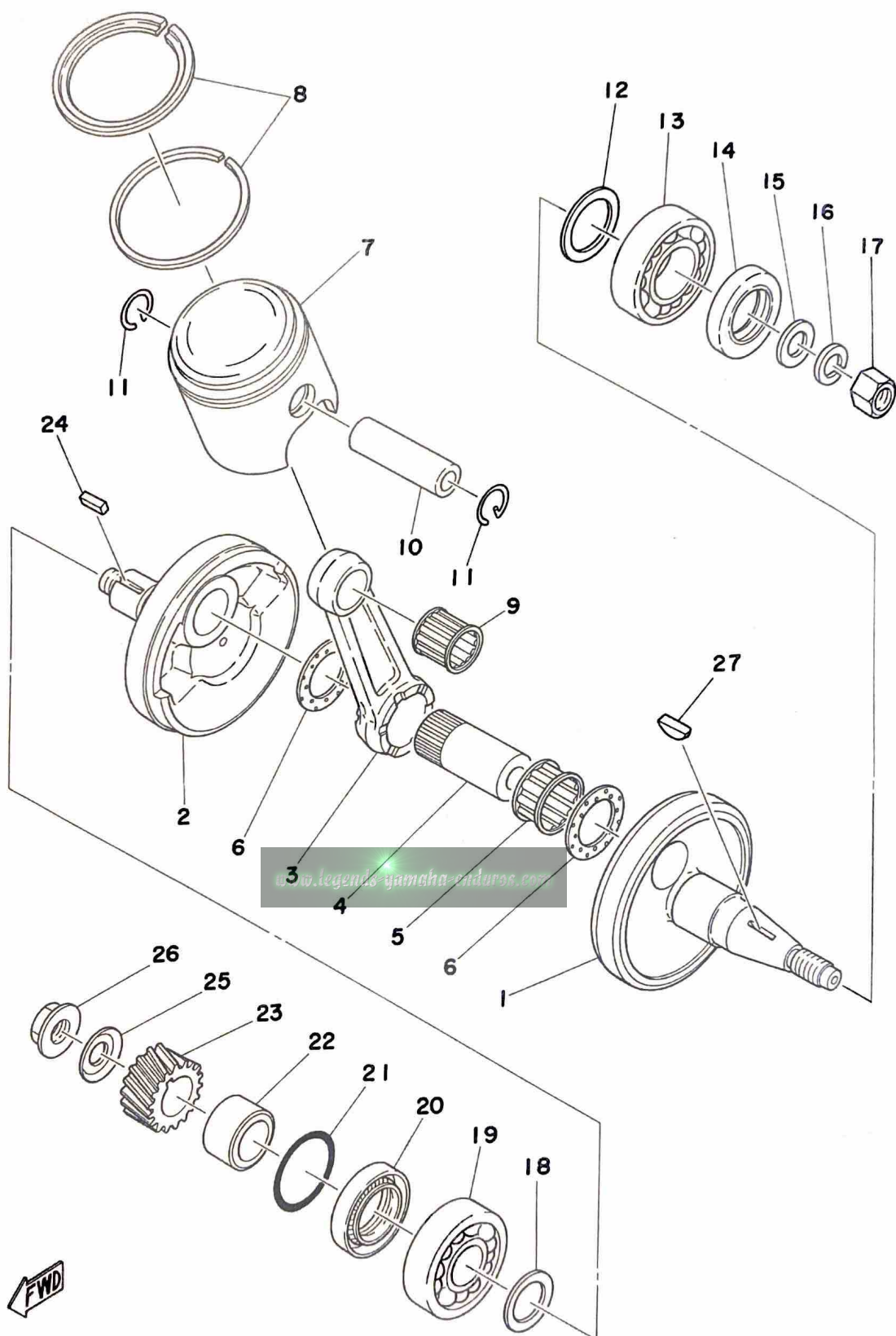
Fig. 4 CRANK · PISTON
