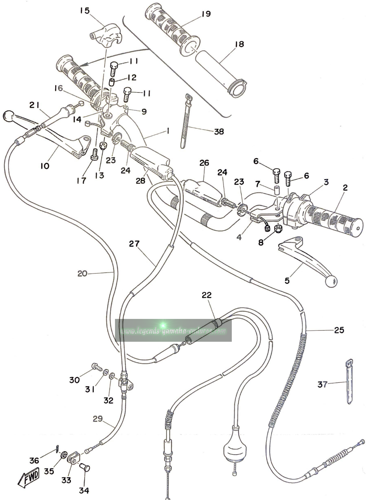
Fig. 21 HANDLE · WIRE
