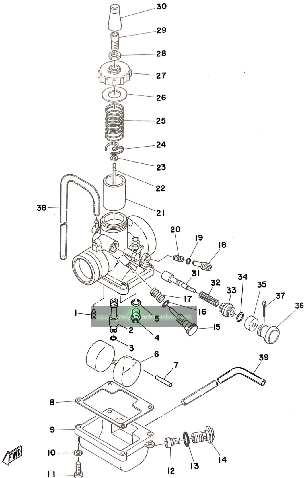
Fig. 11 CARBURETOR
