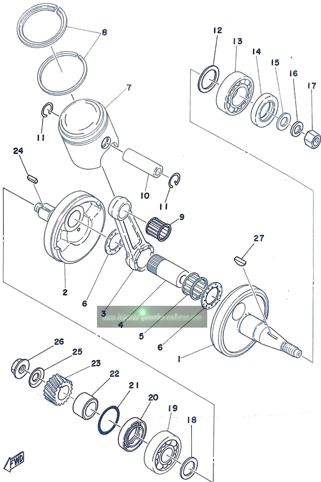
Fig. 4 CRANK · PISTON
