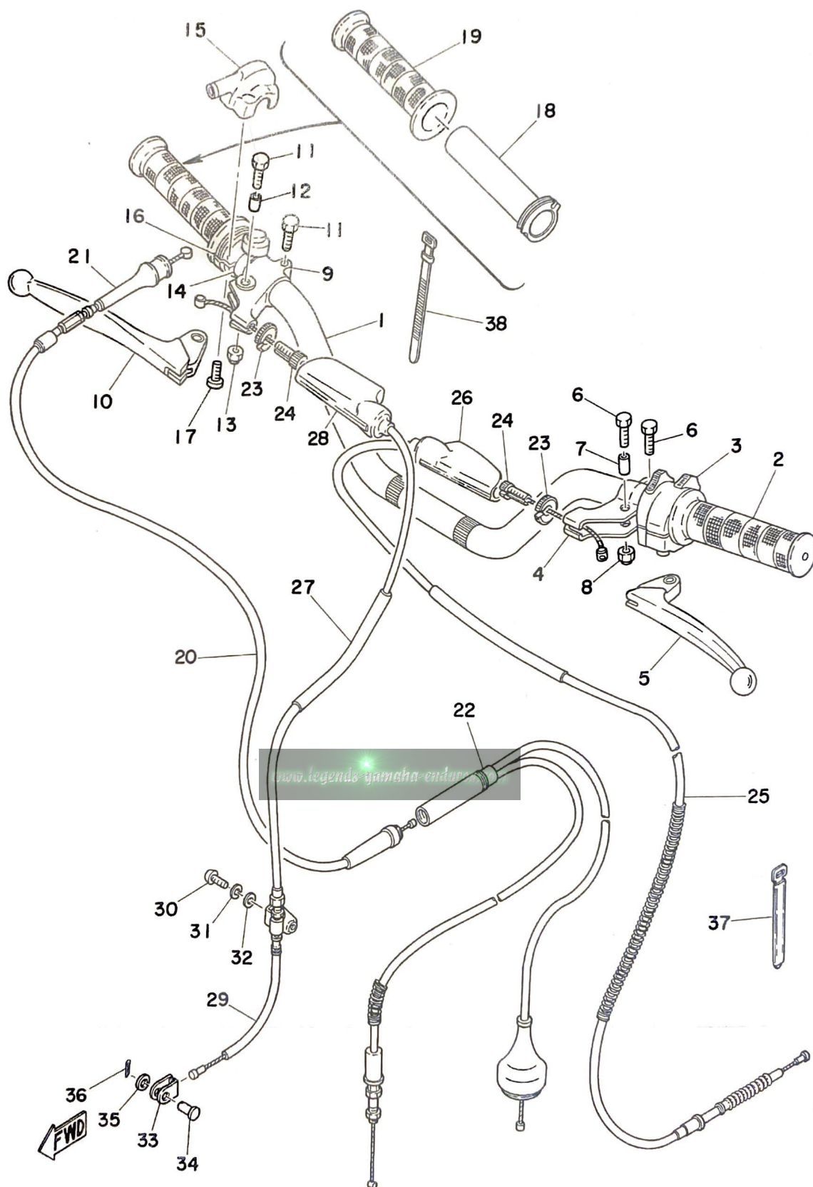
Fig. 21 HANDLE · WIRE
