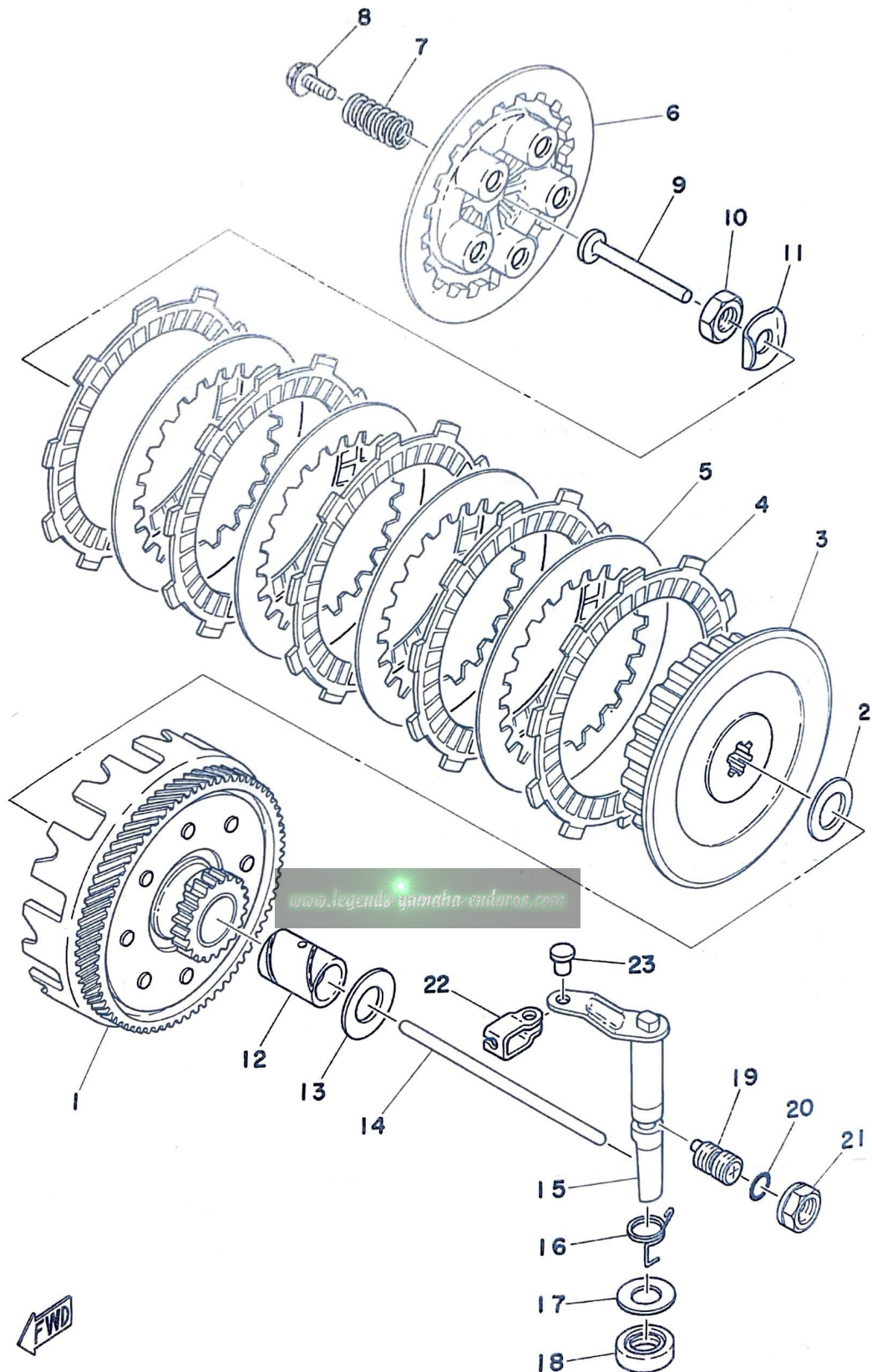
Fig. 5 CLUTCH
