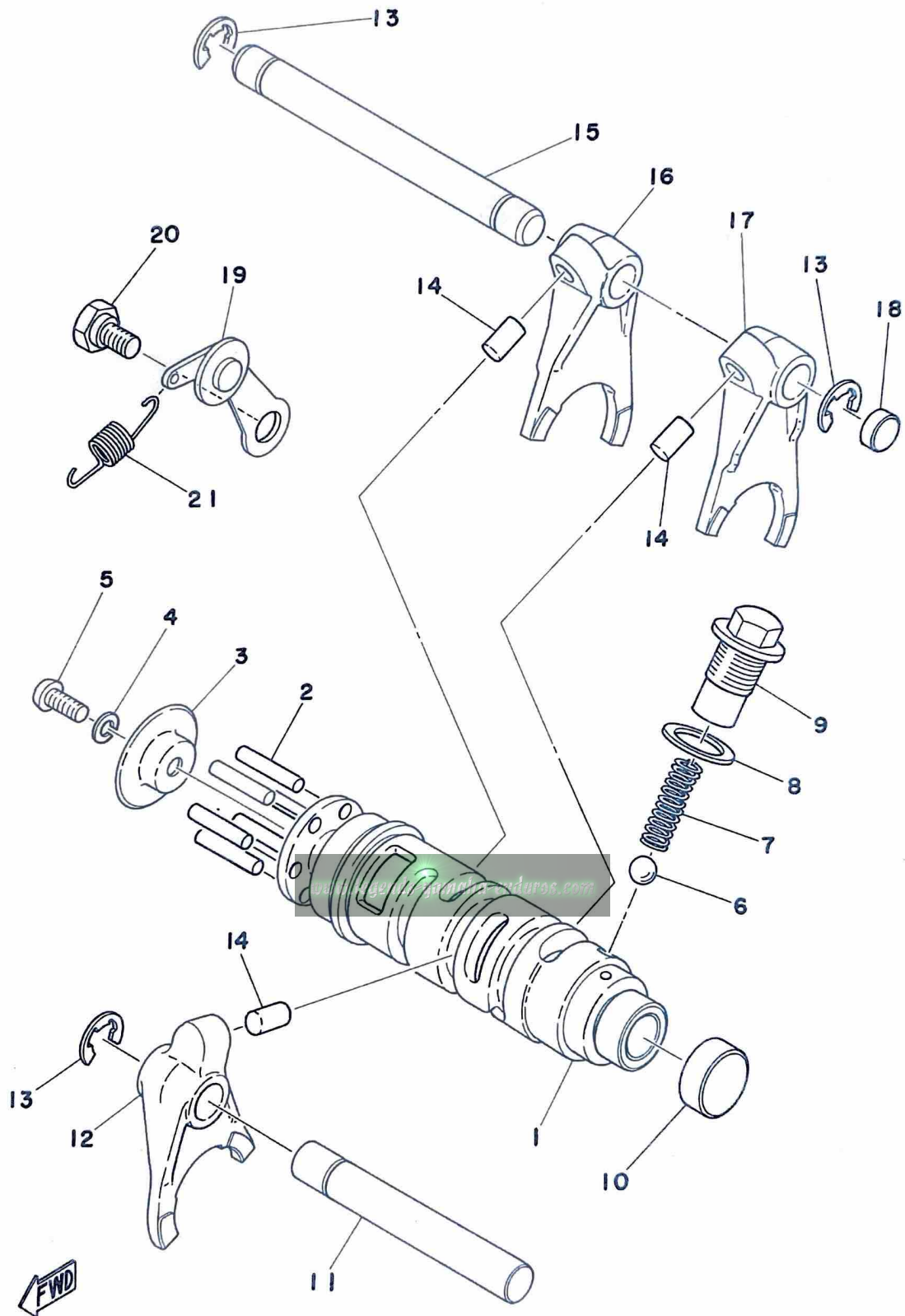
Fig. 7 SHIFTER 1
