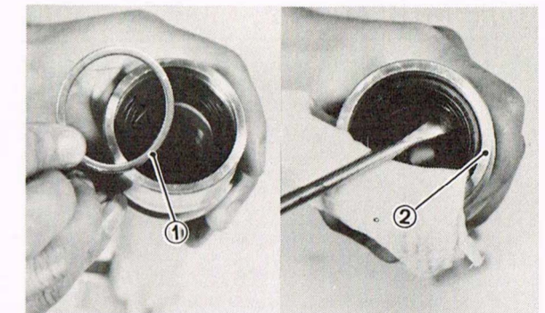
1. Washer 2. Oil seal 1. Rondelle 2. Bague d'étanchéité
