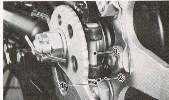
1. Cotter pin 1. Goupille d'assemblage 2. Plain washer 2. Rondelle plate 3. Clevis pin 3. Goupille fendue
