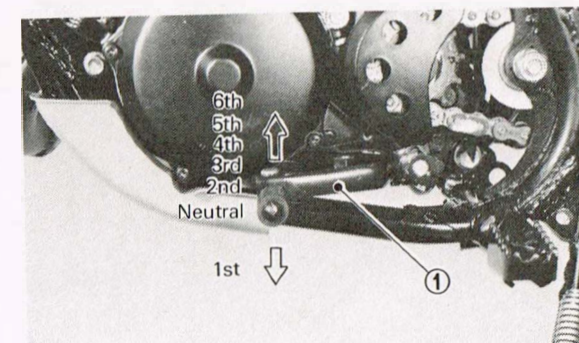
1. Change pedal 1. Pédale de sélecteur de vitesse
