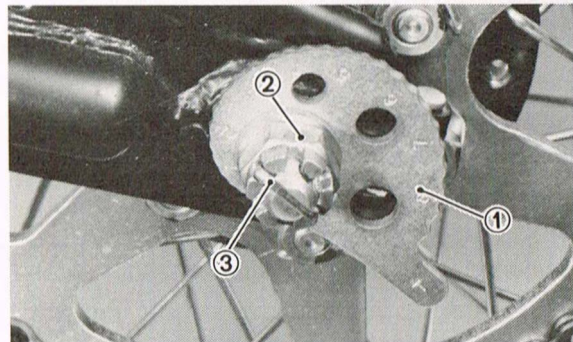
1. Chain puller 1. Tendeur de chaîne 2. Axle nut 2. Ecrou d'axe 3. Cotter pin 3. Goupille
