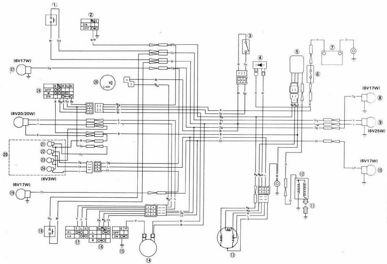
7-3. SCHEMA DE CABLAGE
